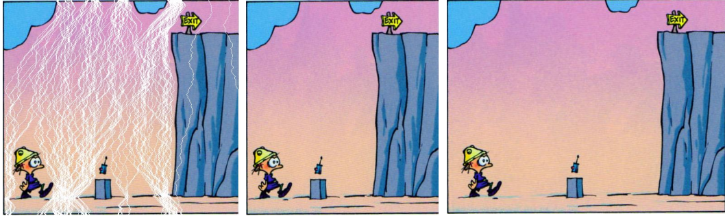
FIGURE 1 – À gauche, l'image de départ où les 100 coutures de coût minimal sont représentées en blanc. Au centre, la version réduite de l'image obtenue en supprimant ces 100 coutures. A droite, la version étendue obtenue en dupliquant ces coutures.
