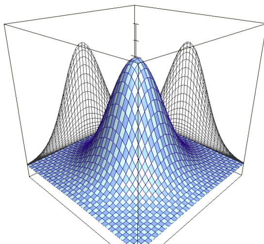
Figure 5.1: Loi normale dans \mathbb{R}^2 avec \mu = (0 \ 0)^T et \Sigma = \text{Diag}(1 \ 1) : f_{\mathcal{X}_1 \mathcal{X}_2}(x_1, x_2) = \frac{1}{2\pi} e^{\left(-\frac{x_1^2 + x_2^2}{2}\right)}
