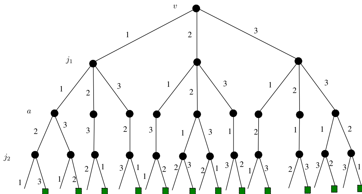
Figure 2.1: Arbres de scénarios pour le jeu du Monty Hall. À la dernière étape, il reste deux possibilités pour le joueur: soit il maintient son premier choix ( j_2 = j_1 ), soit il révisé son choix ( j_2 = \{1, 2, 3\} \setminus \{j_1, a\} ). La politique de décision j_2 qui consiste à systématiquement réviser le choix est indiquée par les feuilles de l'arbre marquées par un carré vert plein. Les scénarios gagnants sont ceux où j_2 = v .
