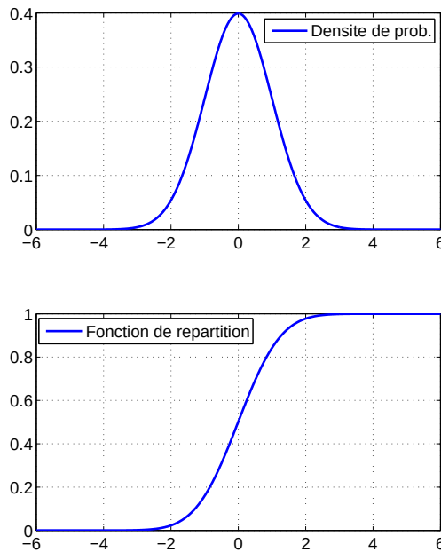
Figure 3.8: (a) Densité de probabilité de la loi normale centrée réduite f_{\mathcal{X}}(x) = \frac{1}{\sqrt{2\pi}} \exp\left(-\frac{x^2}{2}\right) . (b) Fonction de répartition F_{\mathcal{X}}(x) = \int_{-\infty}^x \frac{1}{\sqrt{2\pi}} \exp\left(-\frac{z^2}{2}\right) dz . (Avec le code MATLAB permettant de générer ces courbes).
