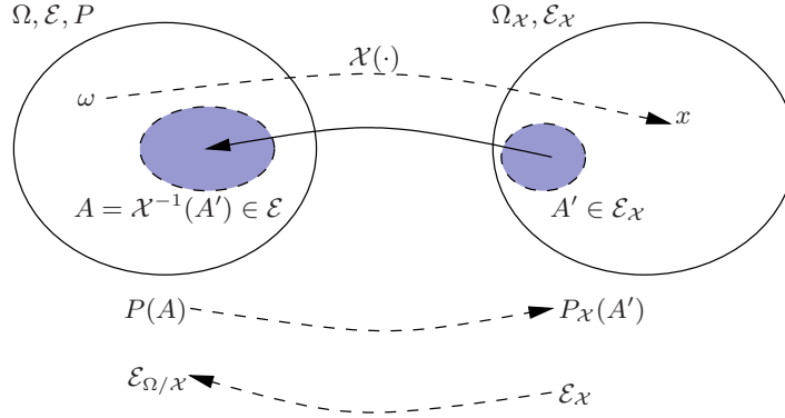
Figure 3.1: Notion de variable aléatoire. On a x \in A' \Leftrightarrow \omega \in A = \mathcal{X}^{-1}(A') , et A' \in \mathcal{E}_{\mathcal{X}} \Rightarrow A \in \mathcal{E} . On a P_{\mathcal{X}}(A') = P(A) . \mathcal{E}_{\Omega/\mathcal{X}} est l'ensemble des parties de \Omega pouvant s'exprimer comme \mathcal{X}^{-1}(A') avec A' \in \mathcal{E}_{\mathcal{X}} .
