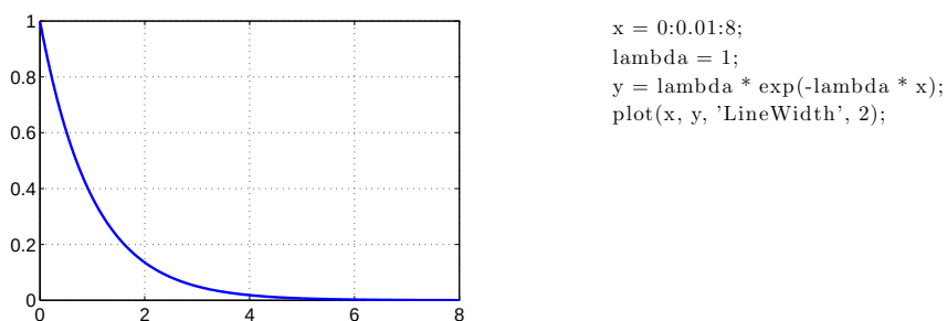
Figure 3.7: Densité de probabilité de la loi exponentielle avec \lambda = 1 , avec le code MATLAB permettant de générer la figure
