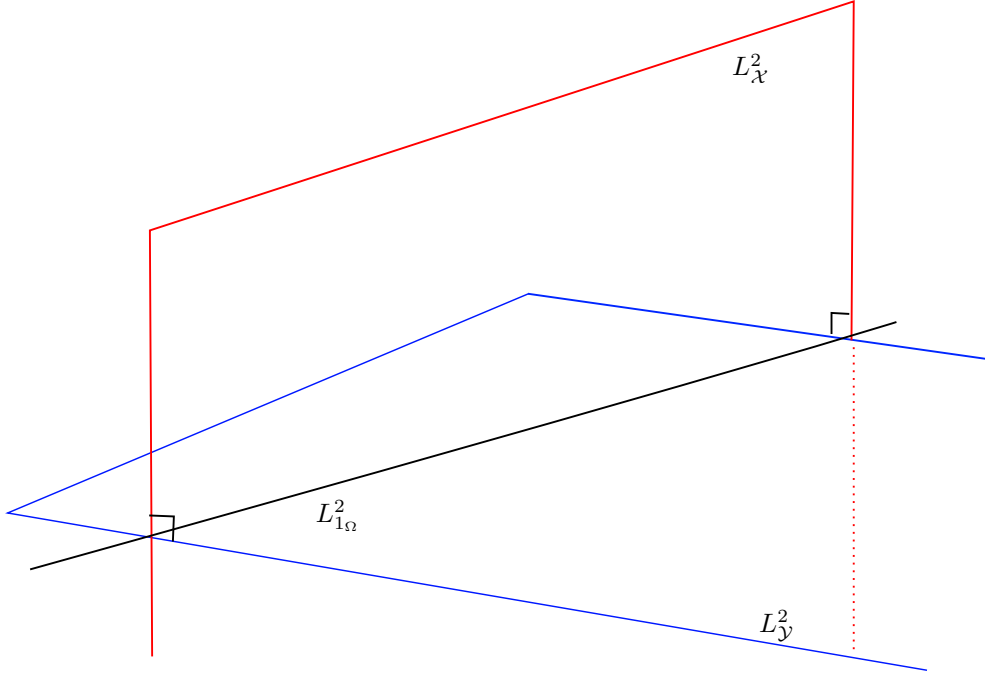
Figure 4.9: Les variables \mathcal{X} et \mathcal{Y} sont indépendantes si et seulement si les espaces de fonctions L^2_{\mathcal{X}} et L^2_{\mathcal{Y}} sont “orthogonaux le long de la droite des constantes L^2_{1\Omega} ”. L^2_{\mathcal{X}} \cap L^2_{\mathcal{Y}} est alors la droite des constantes L^2_{1\Omega} et la projection d’un point de L^2_{\mathcal{X}} sur L^2_{\mathcal{Y}} appartient alors à L^2_{1\Omega} de même que la projection d’un point de L^2_{\mathcal{Y}} sur L^2_{\mathcal{X}} . La projection d’un point \mathcal{Z} de L^2_{\mathcal{X}} sur L^2_{\mathcal{Y}} (et aussi d’un point \mathcal{V} de L^2_{\mathcal{Y}} sur L^2_{\mathcal{X}} ) est donc une v.a. (constante) appartenant à L^2_{1\Omega} et la variable \mathcal{Z} - E\{\mathcal{Z}\} est orthogonale à L^2_{\mathcal{Y}} . Pour tout couple (\mathcal{Z}, \mathcal{V}) \in L^2_{\mathcal{X}} \times L^2_{\mathcal{Y}} on a donc \text{cov}\{\mathcal{Z}; \mathcal{V}\} = 0
