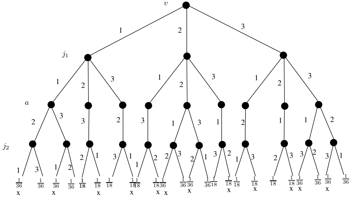
Figure 2.2: Probabilités associées aux feuilles de l'arbre de scénarios pour le jeu du Monty Hall, lorsque le joueur applique la stratégie totalement aléatoire. Les scénarios gagnants sont ceux où j_2 = v , et sont indiqués par des croix. La probabilité de remporter le lot vaut \frac{6}{36} + \frac{6}{18} = \frac{1}{2} .
